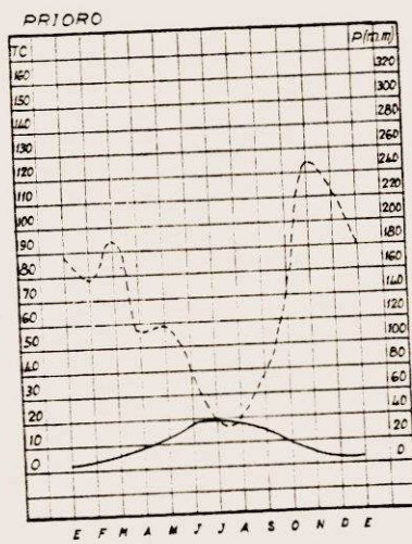
FIG-1 CURVAS PLUVIOTERMICAS
