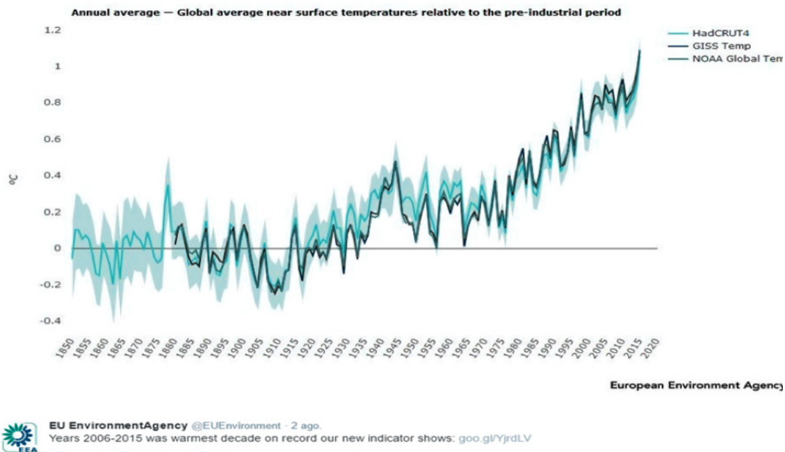
Gráfico 1.4: Temperatura global 1850-2015.
